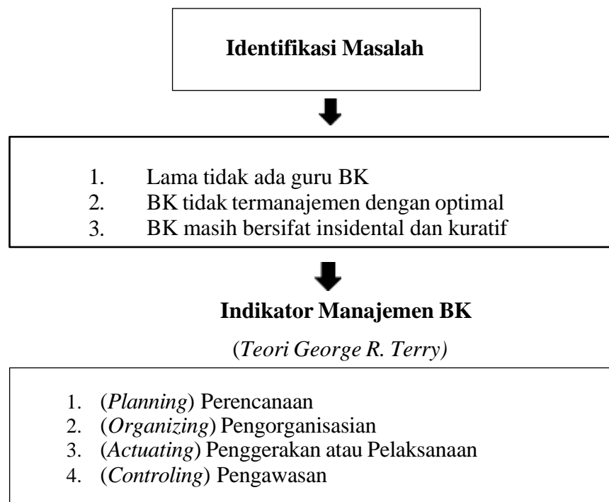
Gambar I Kerangka Teori
