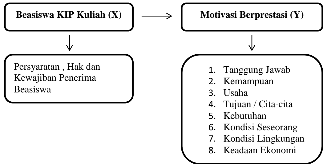
Gambar 1 Kerangka Teori
